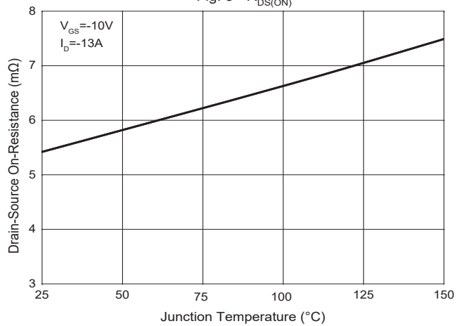
Fig. 5 - R_{DS(ON)}
